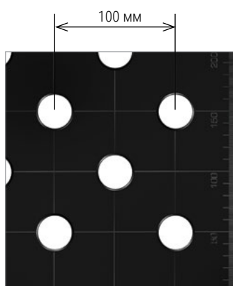
Шаг отверстий — 100x100 мм Дополнительно диагональная сетка отверстий Шаг матричной сетки — 100x100 мм
