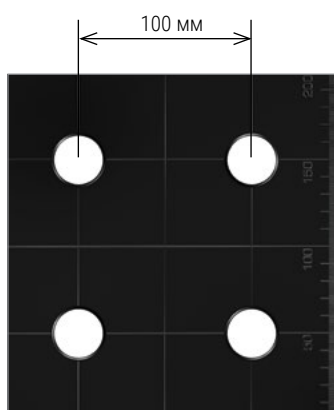
Шаг отверстий — 100x100 мм Шаг матричной сетки — 100x100 мм
